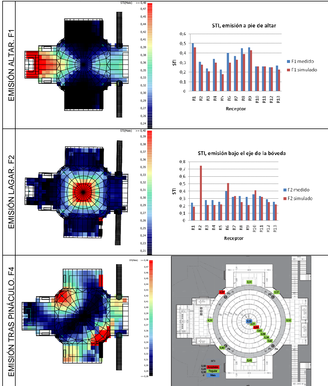
Fig. 6. Comparación STI medidos y simulados.
