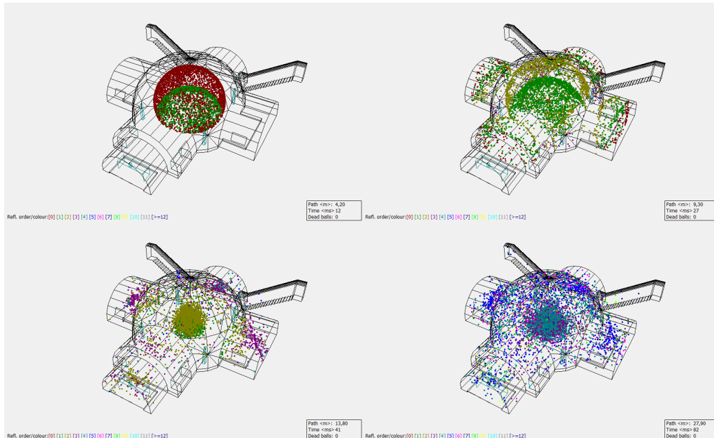
Fig. 5. Propagación del sonido al emitir desde F2.
