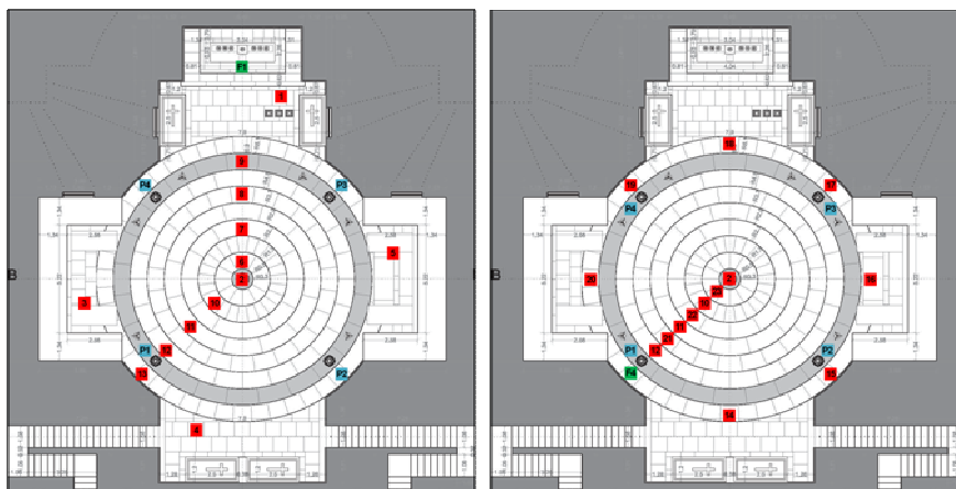
Fig. 3. Distribución de los receptores al emitir desde la posición del oficiante (izquierda) y en la galería de susurros (derecha).
