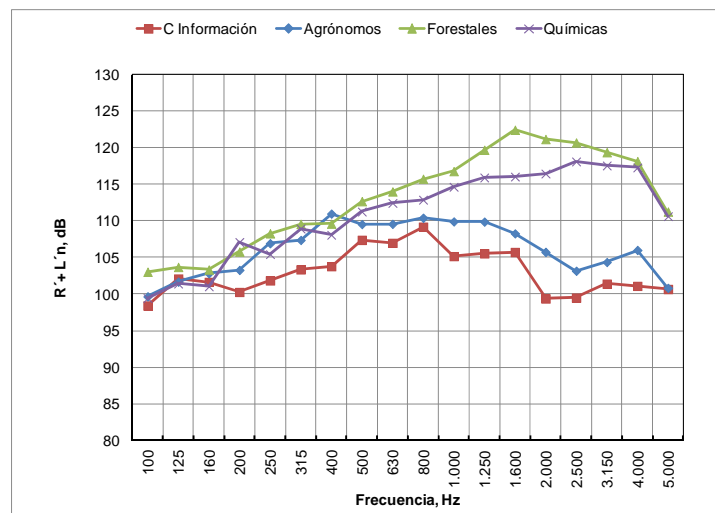
Figura 4. Suma de los valores medidos de R' + L'_n en los recintos objeto de ensayo
