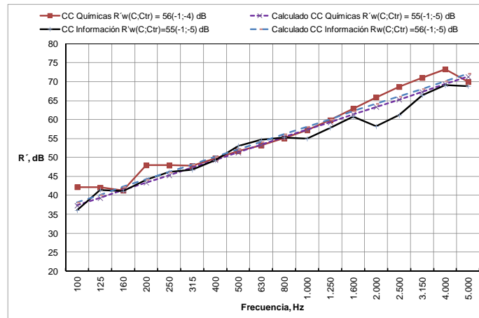
Figura 3. Comparación de los índices de reducción acústica aparentes medidos y calculados.
