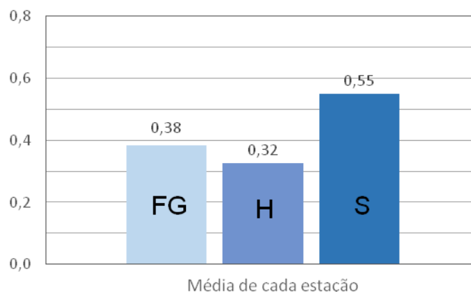
Fig. 6 - Média geral para cada estação (8 posições) das medições do RASTI (FG - Faria Guimarães , H - Heroísmo , S - Salgueiros )
