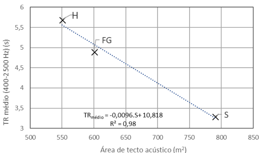
Fig. 9 - Relação entre o TR médio (400-2500 Hz) e as áreas de tecto acústico nas estações (FG - Faria Guimarães , H - Heroísmo , S - Salgueiros )
