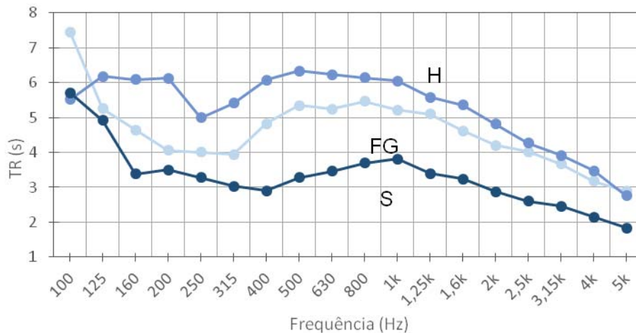
Fig. 7 – Média dos valores do TR das oito medições de cada estação por banda de 1/3 de oitava (FG - Faria Guimarães, H - Heroísmo, S - Salgueiros)
