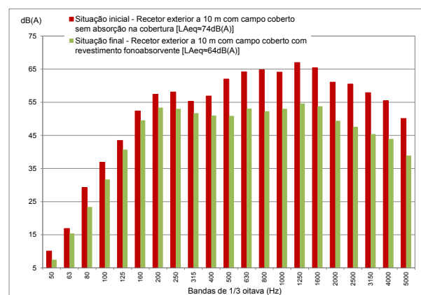
Figura 8. Espectros médios com os níveis sonoros no domínio da frequência e o respetivo valor de LAeq [em dB(A)], obtidos num recetor exterior a 10 m do limite do campo coberto, antes e após intervenção na cobertura.
