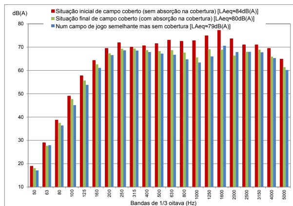
Figura 7. Espectros médios com os níveis sonoros no domínio da frequência e o respetivo valor de LAeq [em dB(A)], obtidos no interior de um campo de jogo coberto, antes e após intervenção, e num outro campo sem cobertura.
