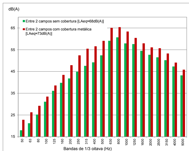
Figura 4. Espectros médios com o níveis de ruído no domínio da frequência e o respetivo valor de LAeq [em dB(A)], obtidos entre dois campos de jogo, com e sem cobertura.
