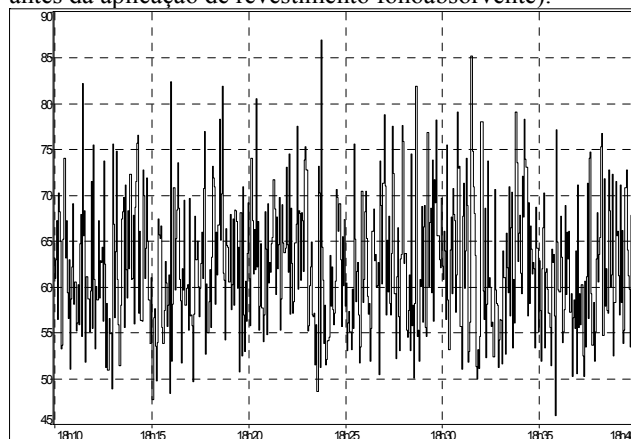
Figura 3. Níveis de ruído “instantâneos” (valores de LAeq para intervalos consecutivos de 3 s), em dB(A), obtidos entre dois campos de jogo sem cobertura.
