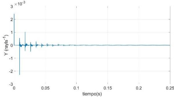
Figura 3. Respuesta al impulso obtenida a partir de la admitancia acústica de un resonador de Helmholtz con pérdidas con una frecuencia de resonancia de 237 Hz conectado a un tubo de 6m de longitud.
