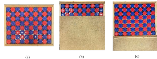
Figura 4. Detalle de algunas configuraciones a estudiar para absorción: (a) Matriz de 10x8 tapones: configuración Plana (P), (b) Matriz con fieltro de cáñamo en parte superior: 0configuración Plana Cáñamo Superior (P-C-S), (c) Matriz con fieltro de cáñamo en parte inferior: configuración Plana Cáñamo Inferior (P-C-I).
