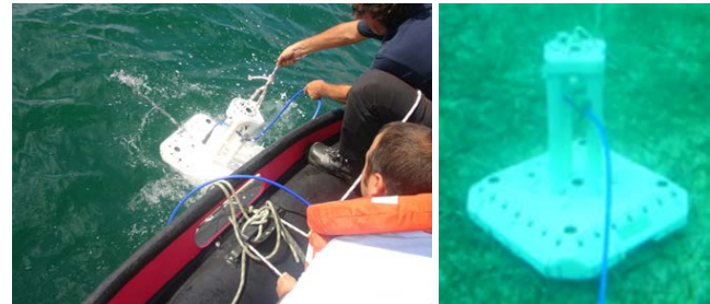
Figura 2. Sensor submarino Multi-Influencia (USU) durante el despliegue (izquierda) y desplegado en el fondo del mar (derecha).
