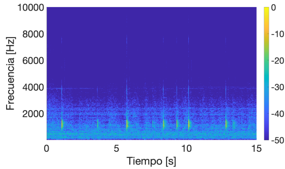
a) Espectrograma de un goteo en presencia de ruido de fondo (ruido de un aspirador doméstico).
