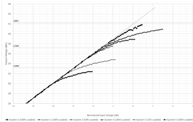
Figura 4. Test lineal STI-PA (sistemas 1-5).
