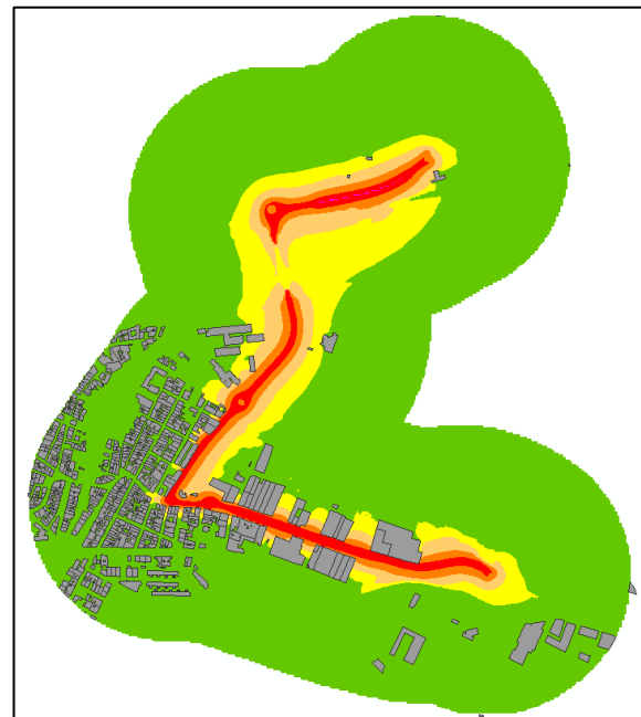
Figura 7: Resultado Lden CNA
