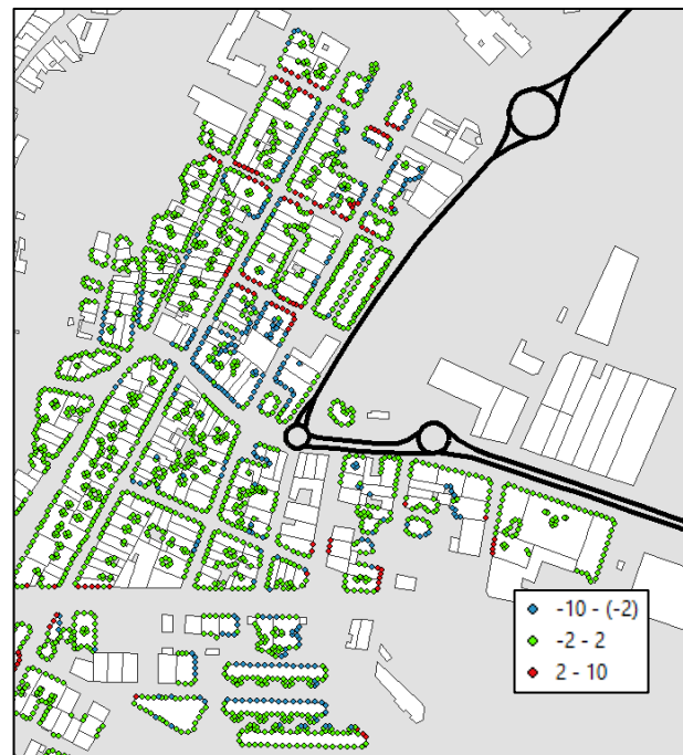
Figura 13: Diferencias en receptores de fachada. Lden
